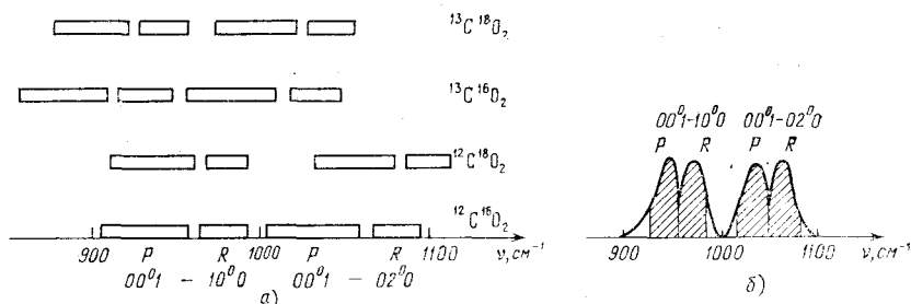
Рис. 16.1. а) Частотные диапазоны дискретной перестройки лазеров на молекулах CO 2 разного изотопического состава. б) Области плавной перестройки CO 2 -лазера (заштрихованы).
