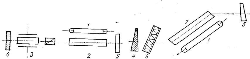
Рис. 20.4. Схема лазера с модулированной добротностью: 1 — лампа накачки, 2 — активный стержень, 3 — модулятор, состоящий из призмы Глана и ячейки Поккельса, 4 — глухое зеркало, 5 — частично прозрачное выходное зеркало.
