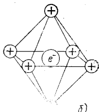
Рис. 23.1. Схема (а) и модель (б) F -центра в ЦГК.
