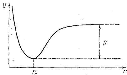
Рис. 15.2. Потенциальная кривая двухатомной молекулы: D — энергия диссоциации, r_e — равновесное расстояние между ядрами.
