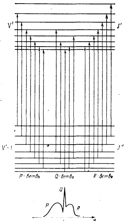
Рис. 15.3. Схема P -, Q - и R -переходов колебательной полосы V' \rightarrow V' - 1 .
