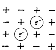
Рис. 23.2. Схема F_2 -центра в ЩГК.
