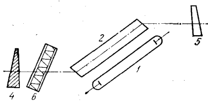
Рис. 20.5. Схема лазера с самосинхронизацией мод (обозначения те же, что и на рис. 20.4). Насыщающий фильтр 6 расположен около левого (глухого) зеркала 4.
