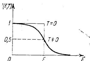
Рис. 24.2. Распределение Ферми ( F — уровень Ферми).
