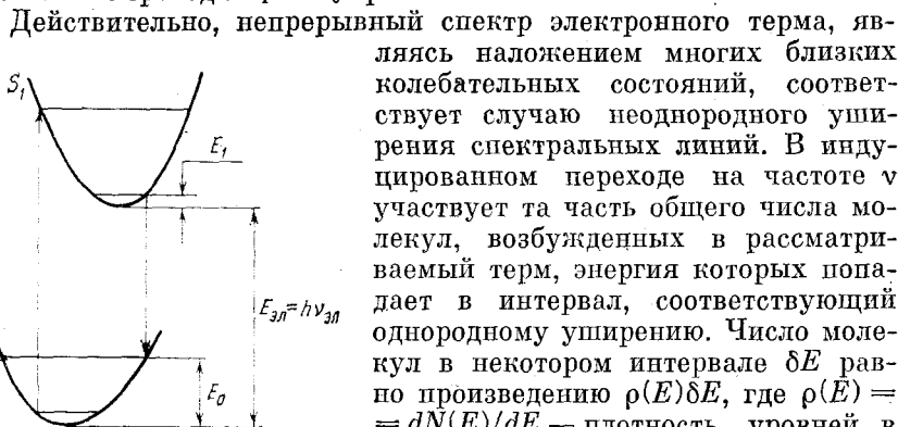
Рис. 22.3. К определению условия положительного усиления.
